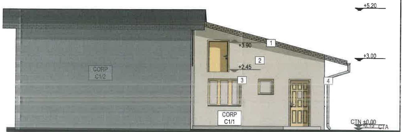
FAȚADĂ PRINCIPALĂ PROPUS CORP C1/1
