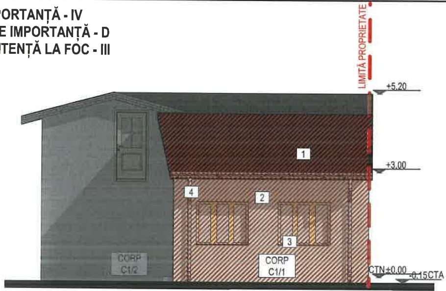
FAȚADĂ SECUNDARĂ PROPUS CORP C1/1
