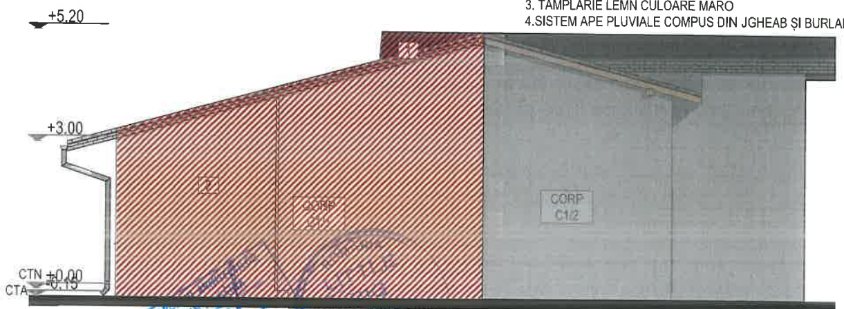
FAȚADĂ POSTERIOARĂ PROPUS CORP C1/1
